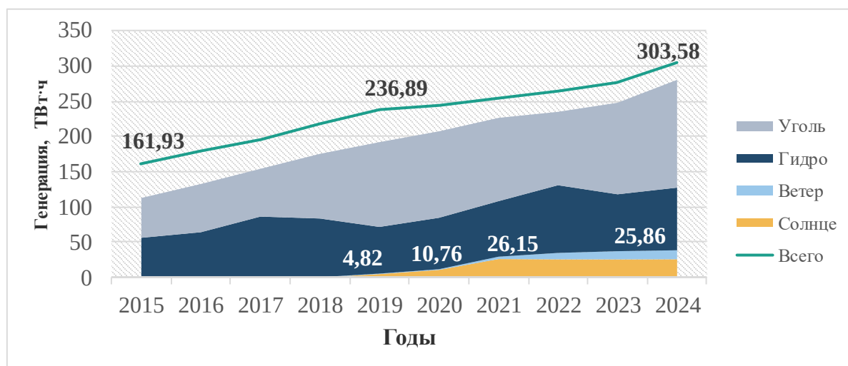
Рис. 2. Генерация электроэнергии во Вьетнаме по видам источника (ТВт·ч) в 2015–2024 гг.
