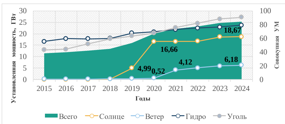
Рис. 1. Установленные мощности во Вьетнаме по видам источника (ГВт) в 2015–2024 гг.
